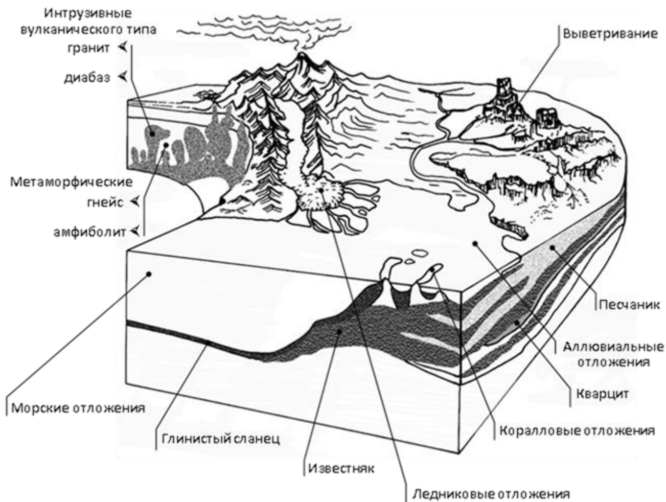
Рис. 1. Расположение горных пород и минералов в литосфере
