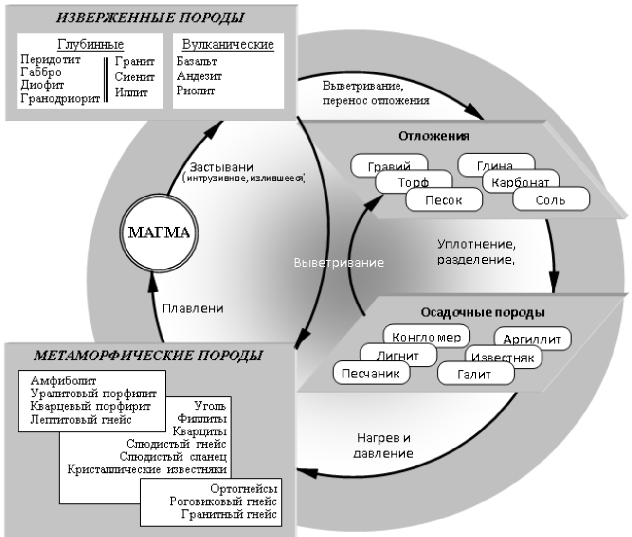
Рис. 2. Схема формирования минералов и горных пород
